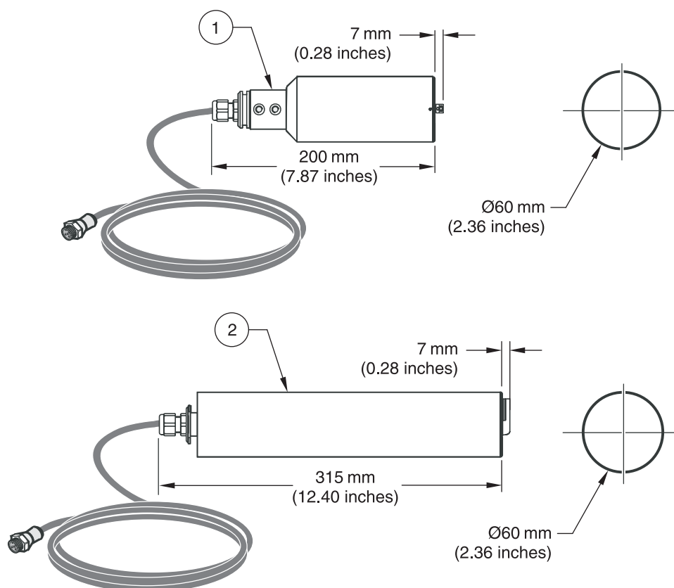
图 2 传感器尺寸
